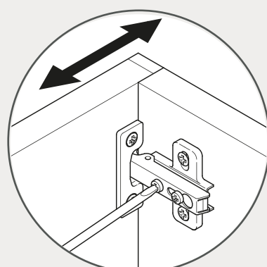
Ajuste lateral
